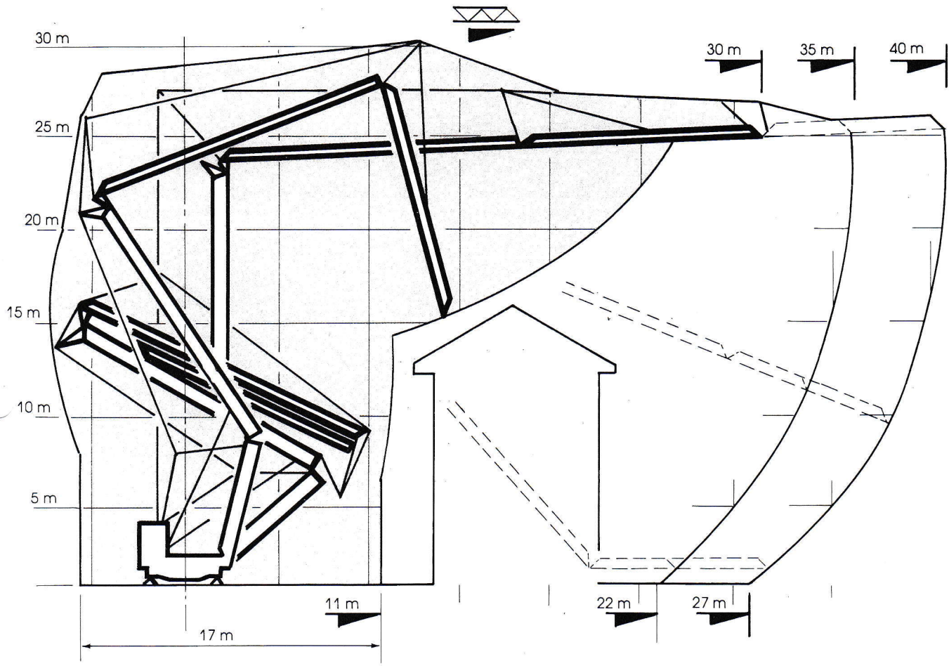
ENCOMBREMENT AU MONTAGE SPACE REQUIREMENT
